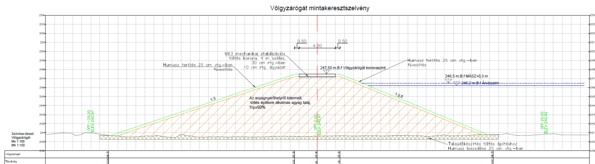
4. ábra: Völgyzárógát mintakeresztmetszelvénye (forrás: VIZITERV Environ Kft.)
